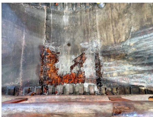
Fig. 7: Afrenset harpiks og genbeskyttelse af syninger.
